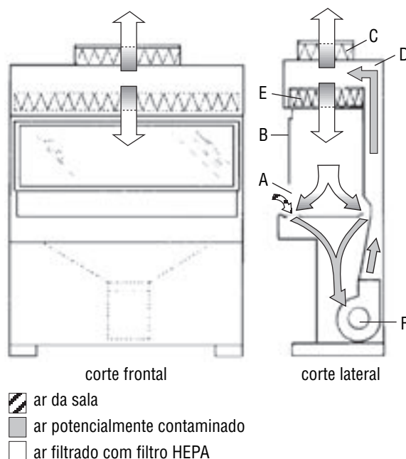
Ilustração 7. Diagrama esquemático de uma câmara de segurança biológica da Classe IIA1 A – Abertura frontal; B – Painel de observação; C – Filtro exaustor HEPA; D – Condução traseira; E – Filtro HEPA de abastecimento; F – Ventoinha
