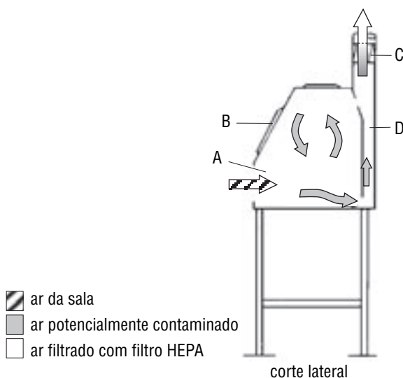
Ilustração 6. Diagrama esquemático de uma câmara de segurança biológica de Classe I A – Abertura frontal; B – Pannel de observação; C – Filtro exaustor HEPA; D – Conduta do exaustor
